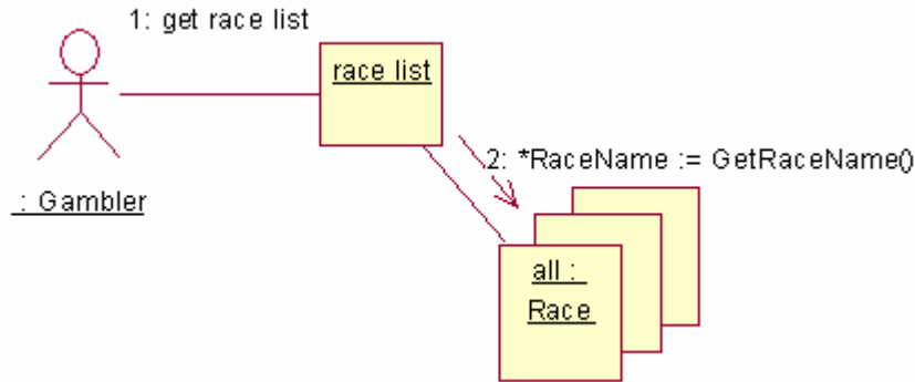
شكل 46: مخطط تعاون
