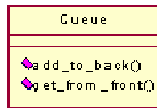
شكل 75: صنفية طابور
